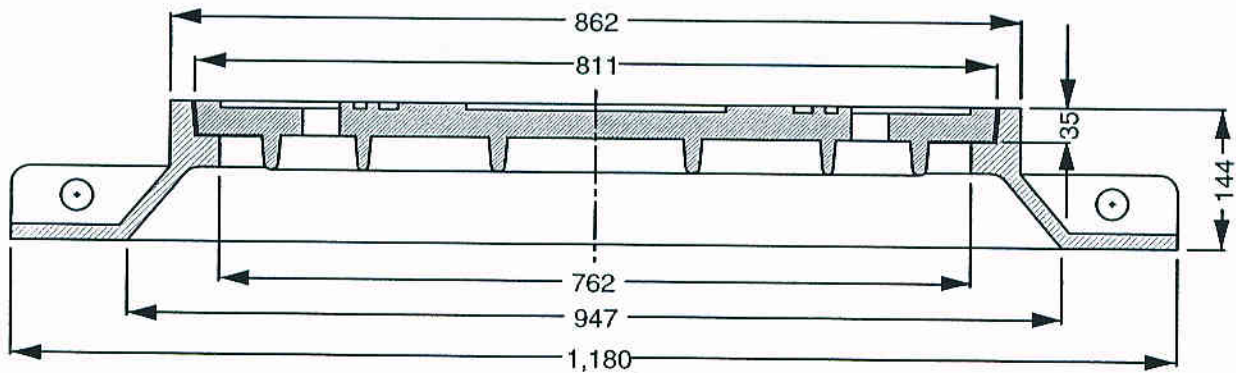
SECTION A-A
