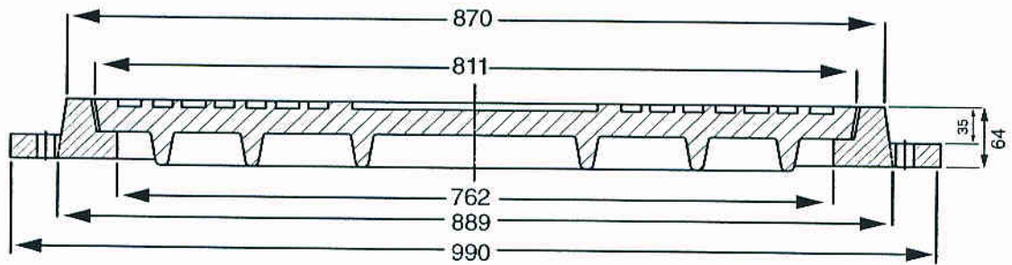
SECTION A-A
